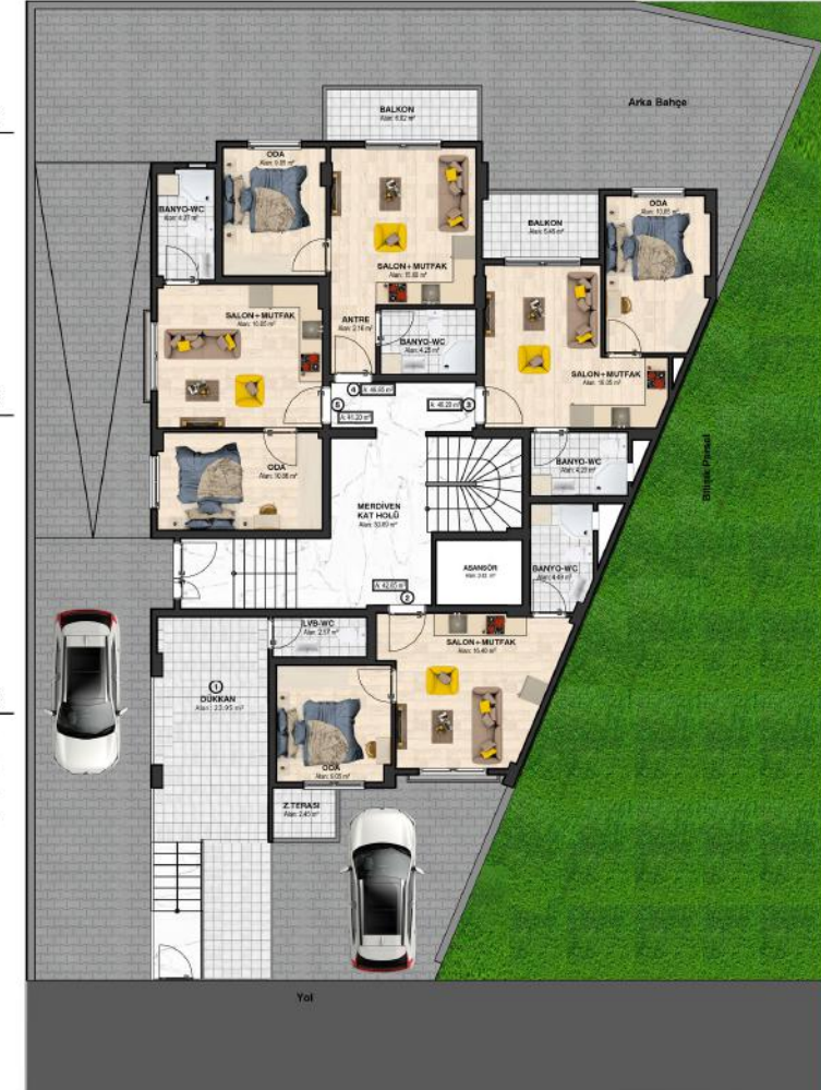
ZEMİN KAT PLANI
