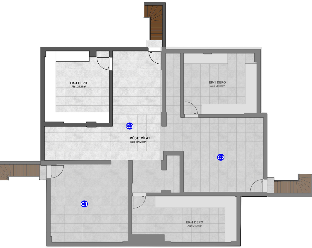
C Blok Bodrum Kat Planı
