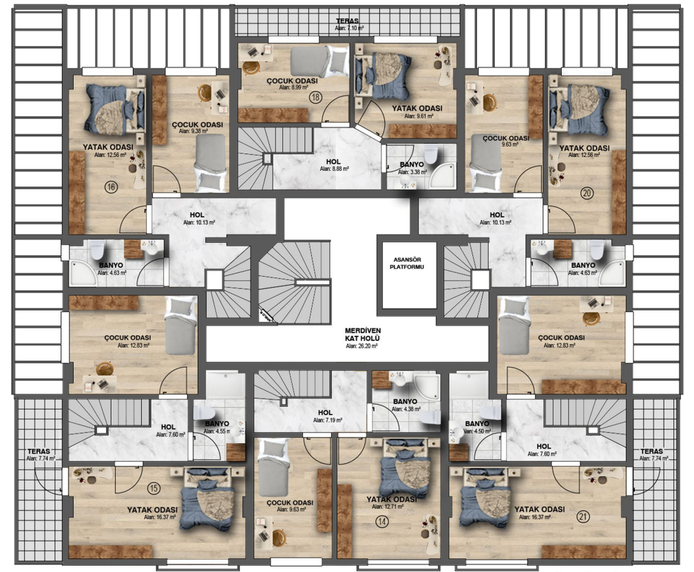
C BLOK ÇATI KATI
